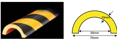
Type R50 - Autocollant
