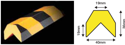
Type AA - Autocollant
