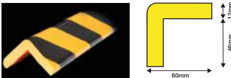
Type H+ - Autocollant
