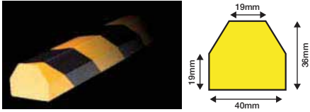
Type CC - Autocollant
