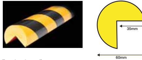
Type A+ - Autocollant
