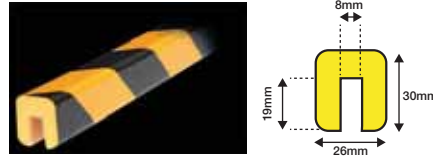
Type G - Autocollant
